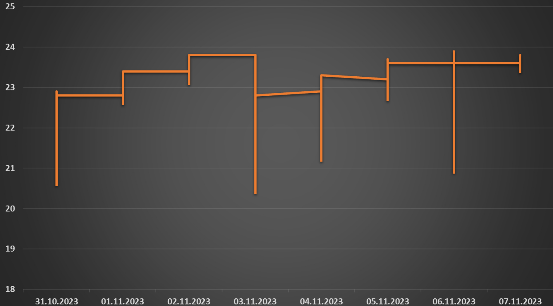
Temperaturverlauf | 31.10.-7.11.2023 | Raum 202
