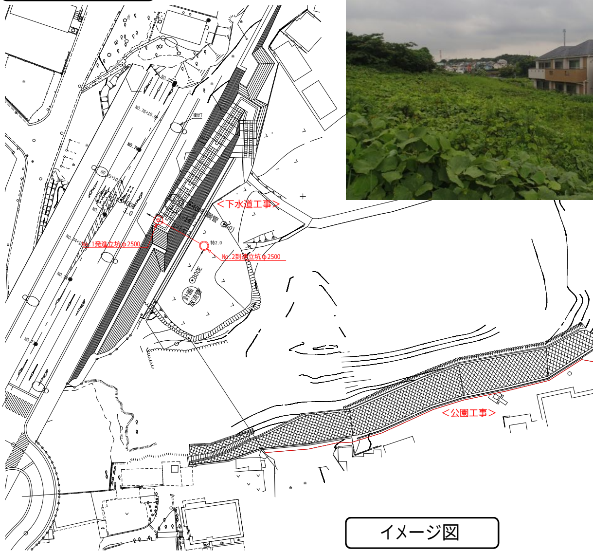
施工平面図
