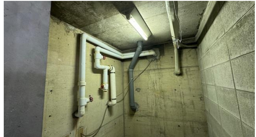
ボイラー室
