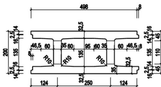
Draufsicht Normalstein
