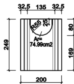
Seitenansicht Eckstein
