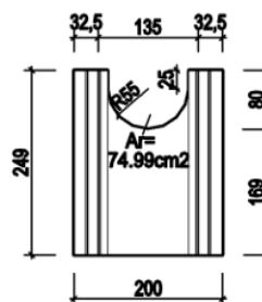
Seitenansicht Normalstein
