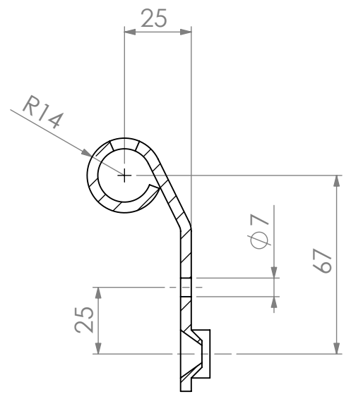
SEZIONE A-A
