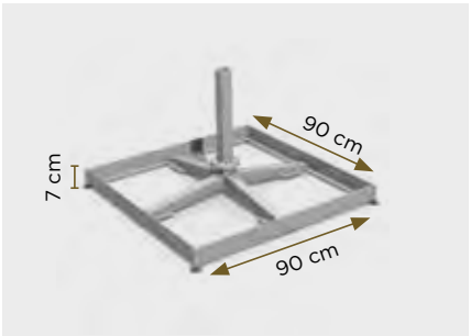
Schirmsockel aus Stahl Mit 8 Fliesen: 130 kg Mit 12 Fliesen: 185 kg Ohne Fliesen
