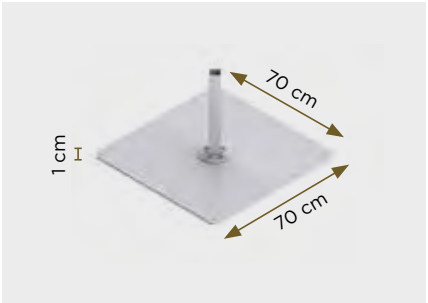
Bodensockel muss chemisch verankert sein. Gewicht: 45 kg
