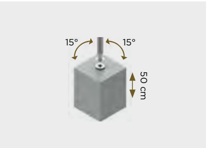
Verstellbare Bodenhülse. Diese Bodenhülse hilft Ihnen mehrere Schirme auf einer geraden Linie zu installieren. Diese Bodehülse gibt Ihnen einen Freidum von bis zu 15° links und auf den rechten Seite
