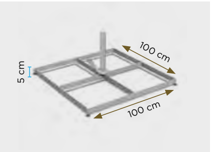
Schirmsockel aus Stahl Mit 4 Fliesen: 115 kg Mit 8 Fliesen: 215 kg Ohne Fliesen
