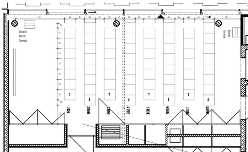
Reihenbestuhlung 60 Sitzplätze
