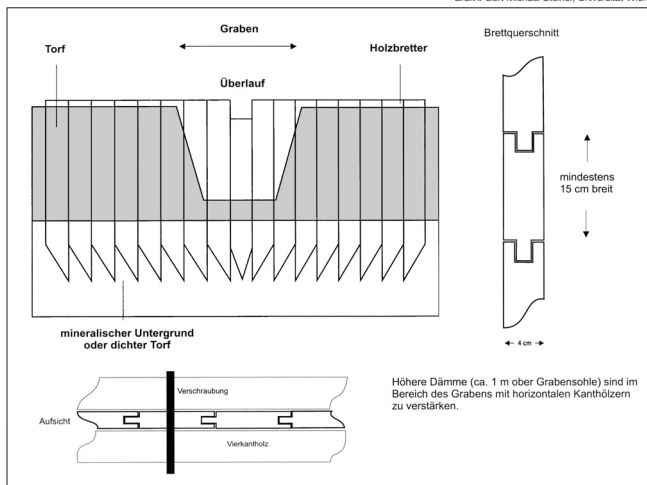
Konstruktionsplan eines Holzdamms
