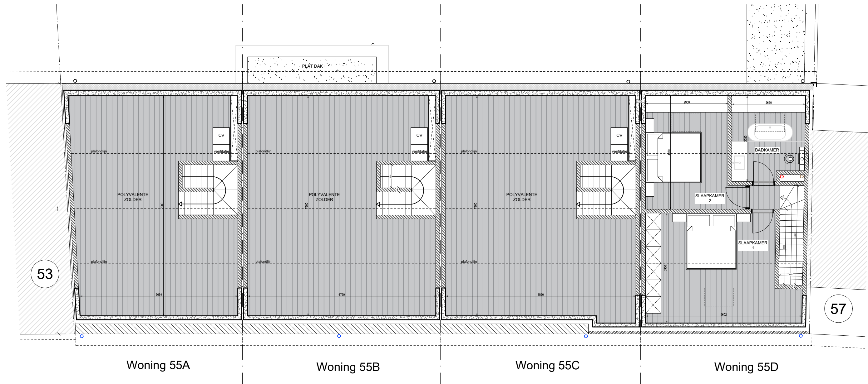
PLAN TWEEDE VERDIEPING
