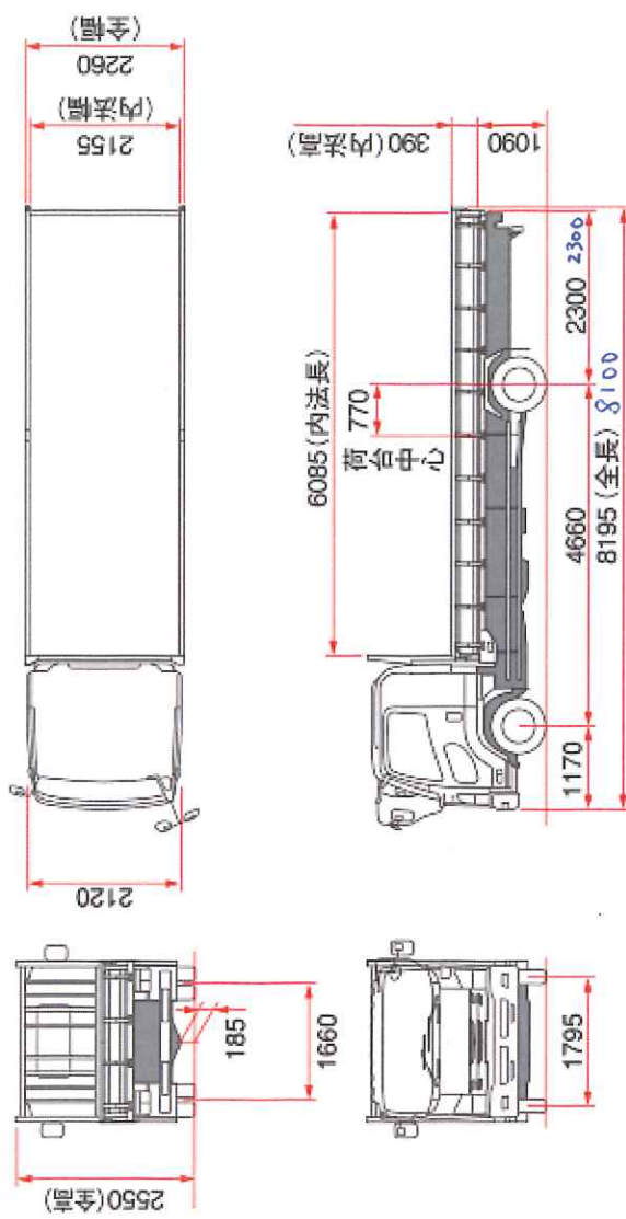
■ 車両外観図
