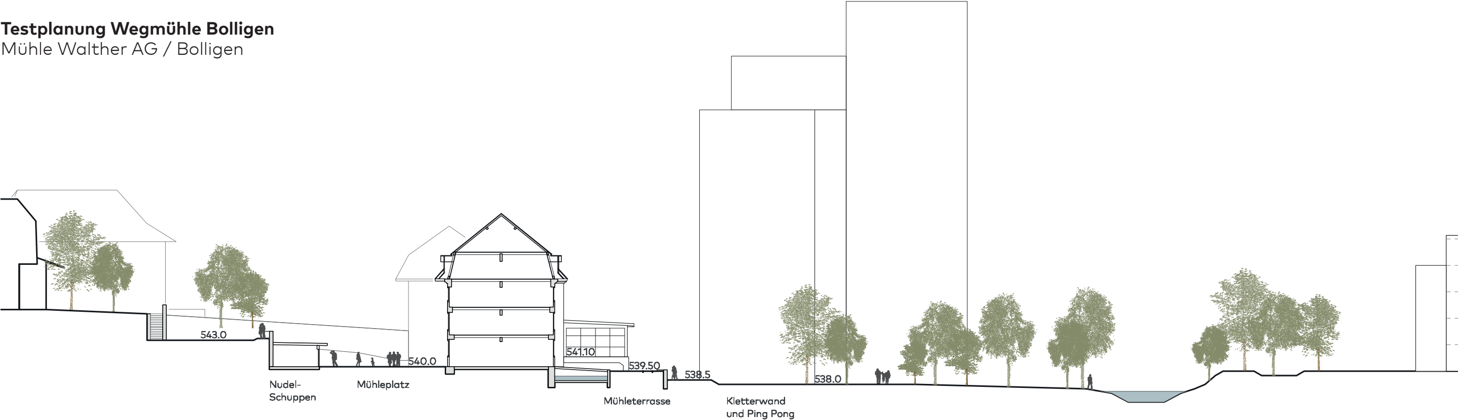
Querschnitt Mühle
