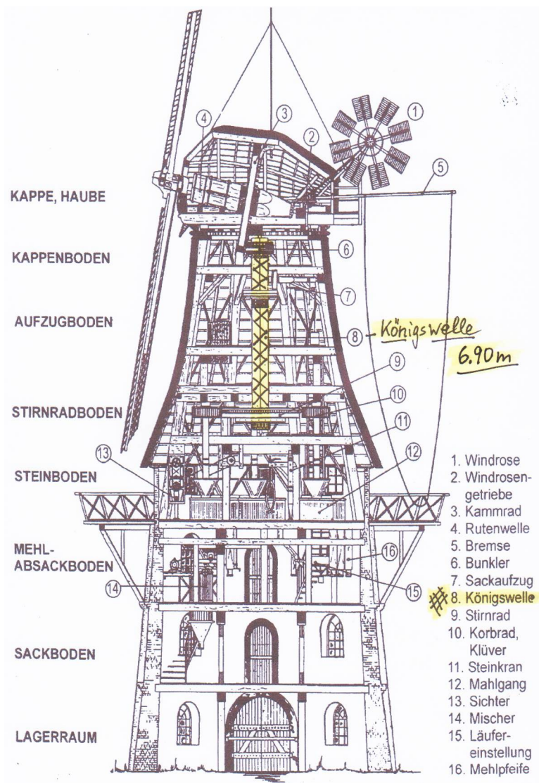
Aufriss der Schiffdorfer Mühle
