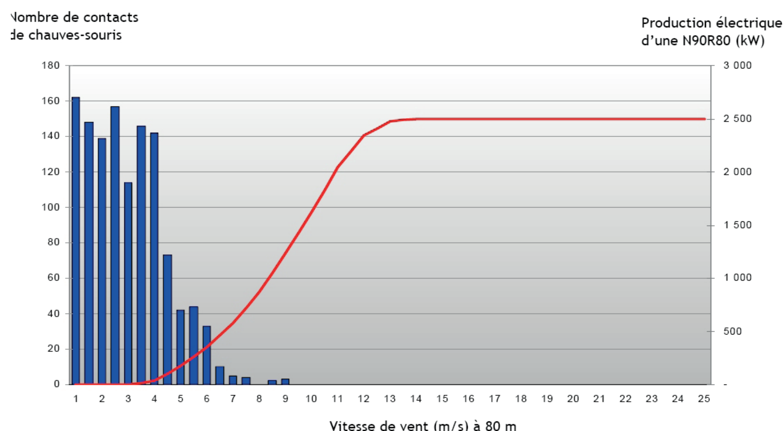
Niveaux d'activité des chauves-souris observés en fonction des vitesses de vent à 80 m de haut.
