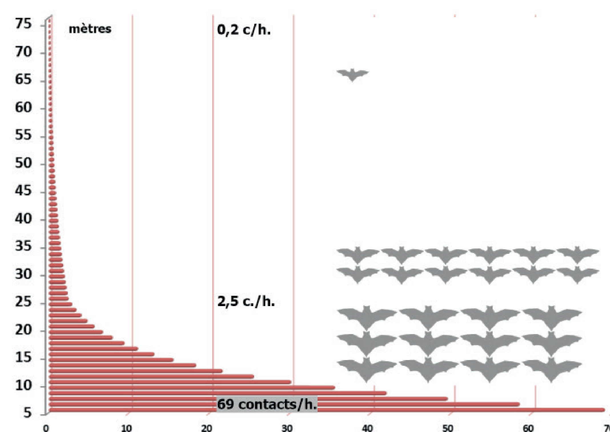
Activité des chauves-souris (en nombre de contacts par heure) en fonction de la hauteur sur un site de projet RES en Haute-Saône
