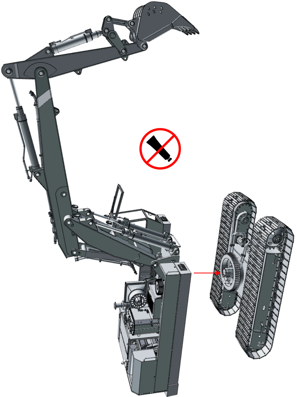
Ober- und Unterwagen
