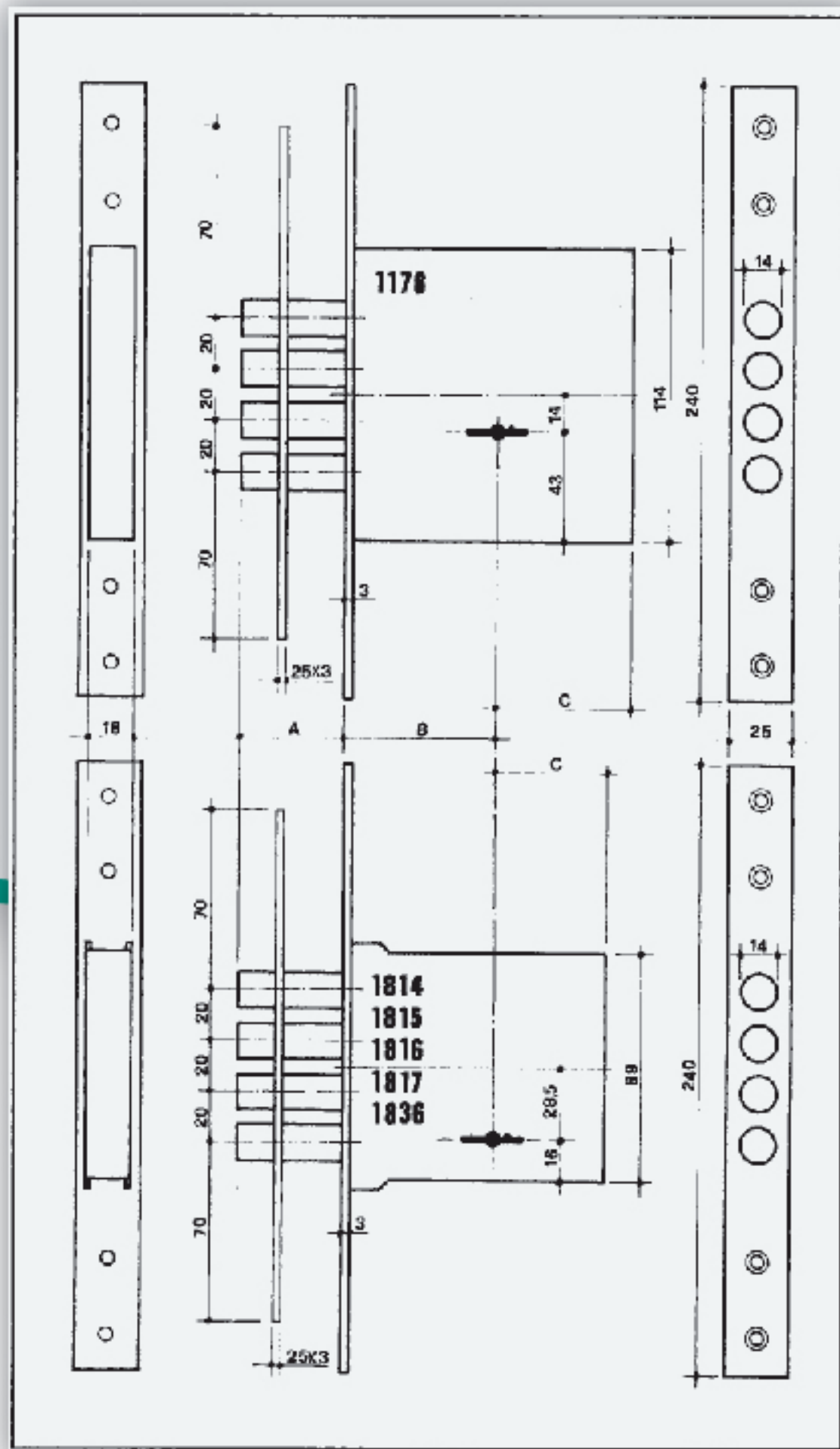
8 LEVE ANTIMANIPOLAZIONE 8-levers, antimanipulation
