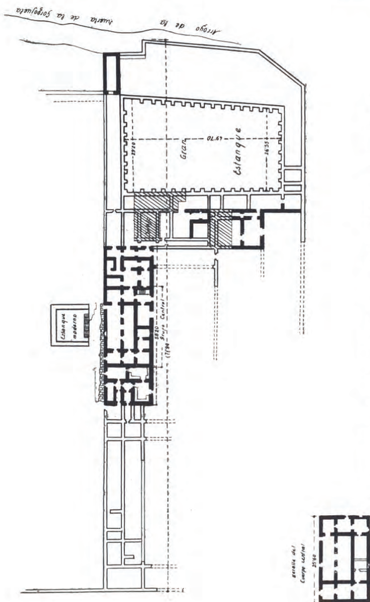
Planta principal del palacio de Almirante, excavado por Velázquez Bosco en 1910
