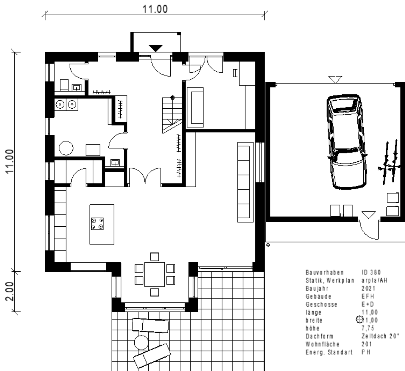
ERDGESCHOSS
