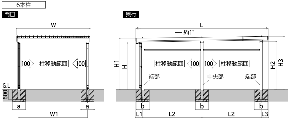
■寸法表
