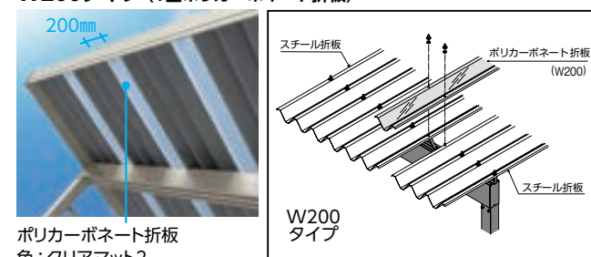
ポリカーボネート折板 色: クリアマット2
