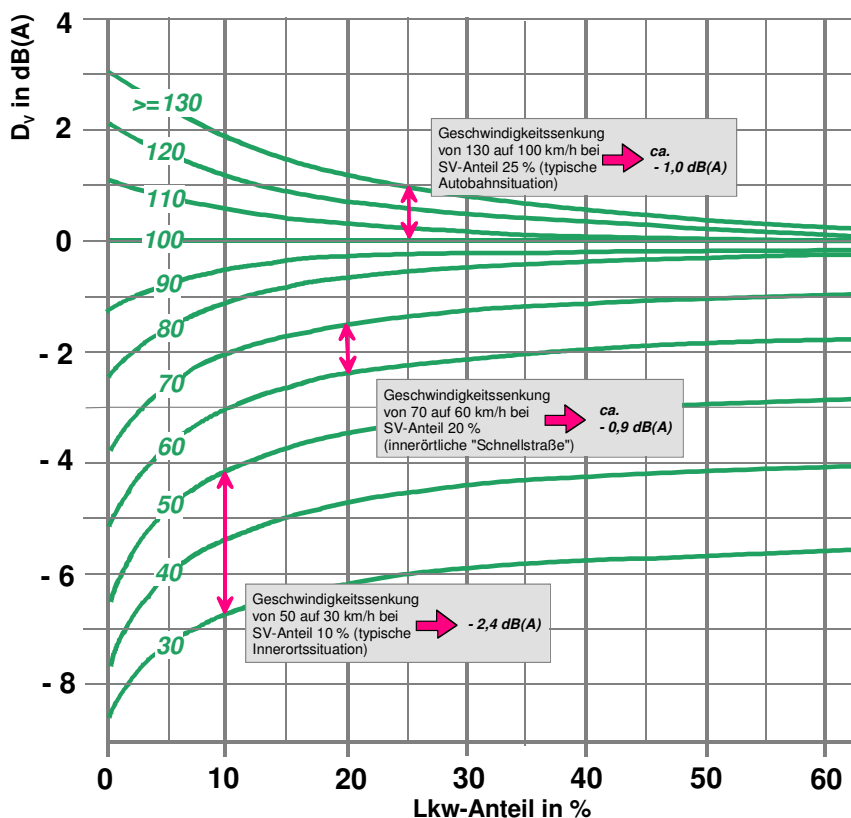
Grafik 6: Zusammenhang zwischen Geschwindigkeit und Schallemissionen (eigene Darstellung auf Grundlage der RLS 90)
