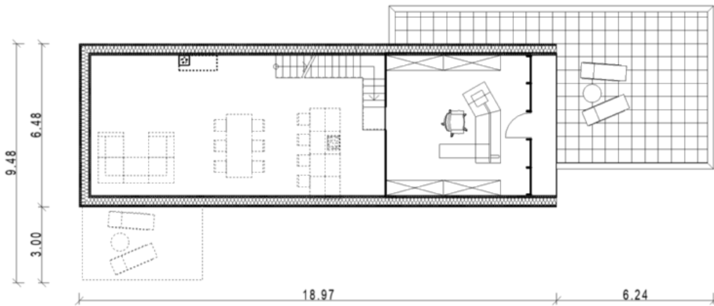
ERDGESCHOSS - OBERGESCHOSS
