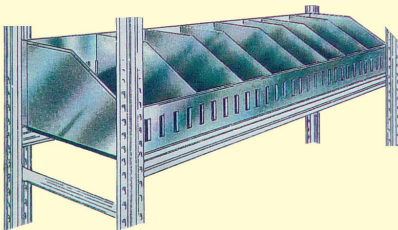
Bordwände H=10cm vorne/H=20 cm hinten
